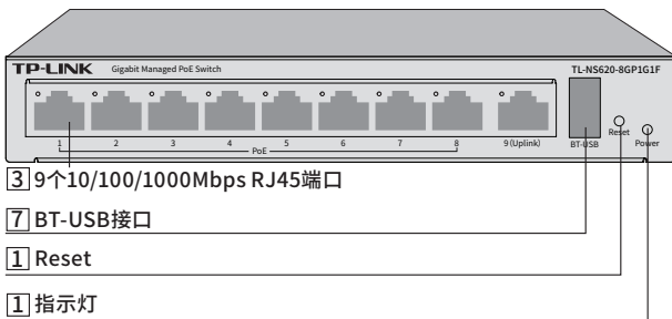
图1-4 TL-NS620-8GP1G1F前面板示意图
