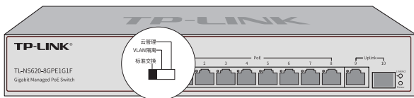
图1-6 系统模式选择开关示意图
