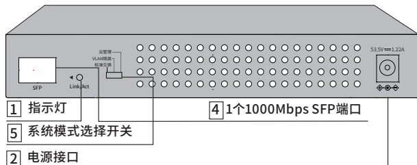
图1-5 TL-NS620-8GP1G1F后面板示意图
