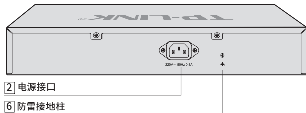
图1-3 TL-NS620-8GPE1G1F后面板示意图
