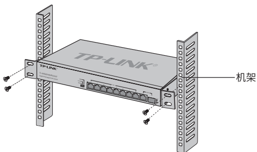
图2-3 机架安装示意图
