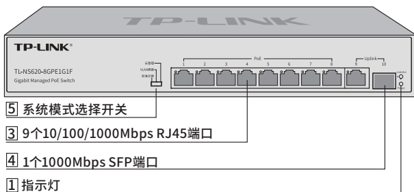
图1-2 TL-NS620-8GPE1G1F前面板示意图
